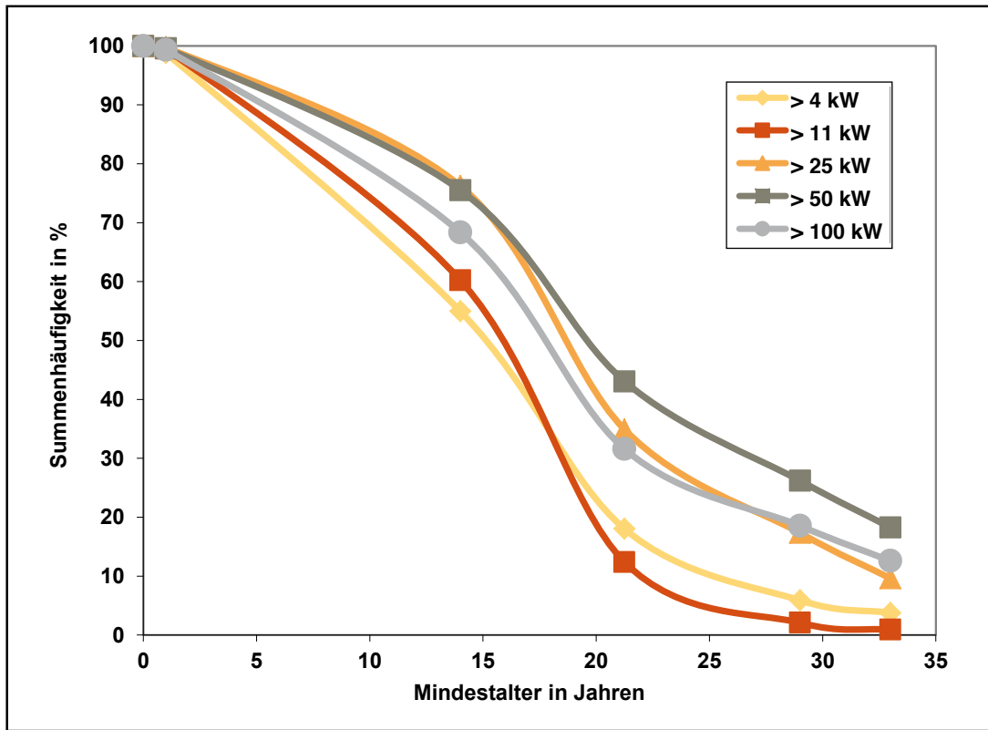
Alterstruktur der Ölfeuerungsanlagen in Deutschland 2011 (Bild 2)
